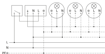
Diagrama electrónico lámpara sin conductor neutro
