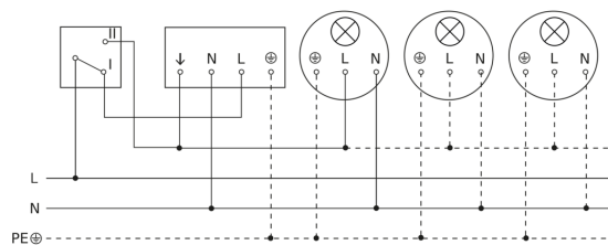
Diagrama electrónico conexión mediante un selector para funcionamiento de alumbrado permanente y automático
